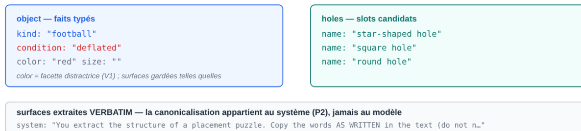
Figure F1 — un épisode réel (mémoire durable, rejouable) : la prose paraphrasée par le modèle, annotée, et son extraction typée verbatim — la sorte, la condition défaisable, la facette distractive, les trous.
