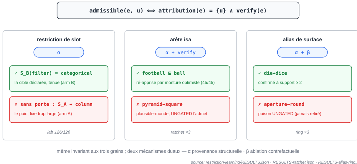
Figure F5 — la porte aux trois grains : le même prédicat d’admission, avec pour chaque grain une unité réellement admise et une unité réellement refusée dans nos runs — la coupe tenue par le bras B contre la dérive du bras A (lab), l’arête ré-apprise contre pyramid→square (cliquet), l’alias confirmé die→dice contre le poison aperture→round (ring, §6.6).
